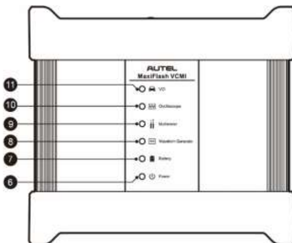
Рисунок 2-6. Устройство VCMi (вид спереди)
